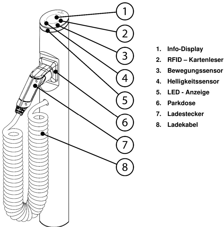
Bedienelemente der electrify Ladesäule eSat
