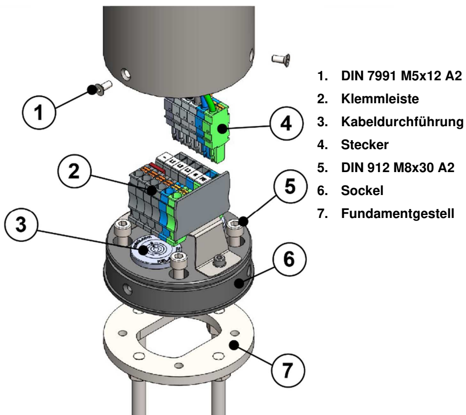
Montage in Kombination mit Fundamentgestell
