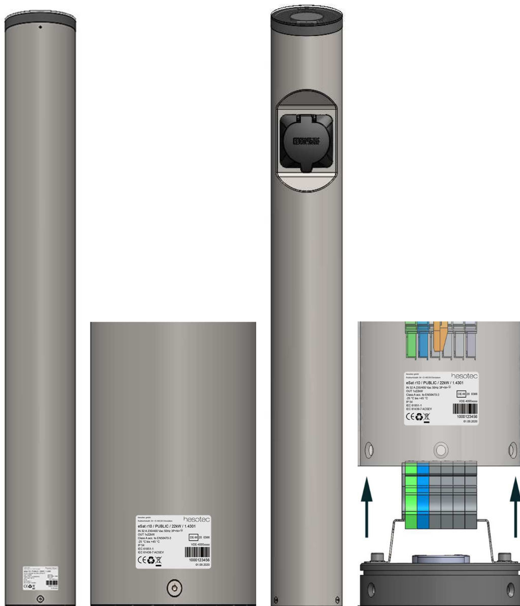
Position Typenschild: 1x Außen und 1x Kopie Innen im Gehäuse
