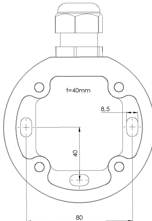
Abmessung der Bohrungspunkte (Maßeinheit mm)
