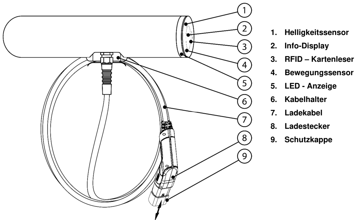
Bedienelemente der electrify eBox wr30
