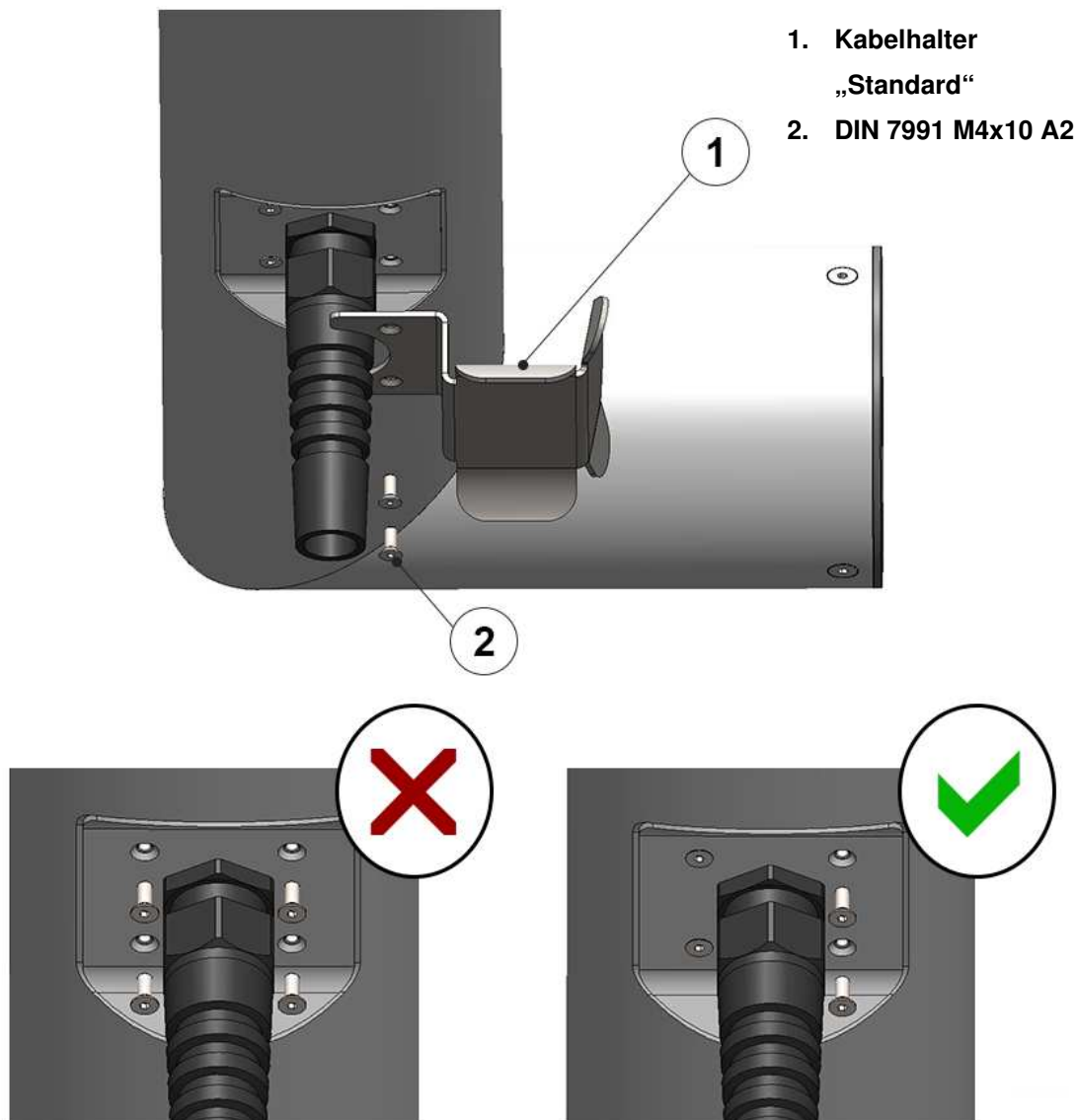
Montagebeispiel des Kabelhalters (innen)
