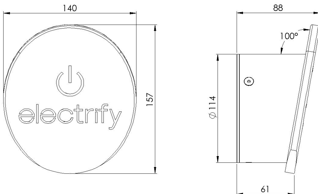
Kabelwandhalter: Abmessung (Maßeinheit mm)
