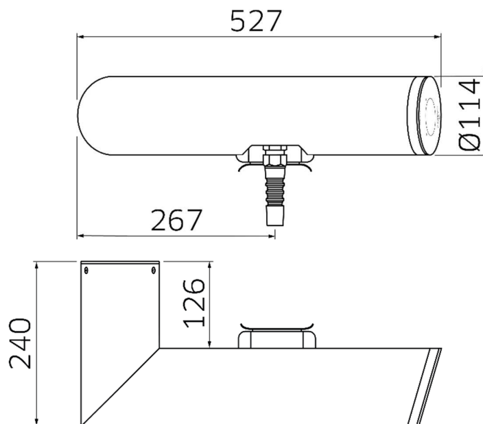
electrify eBox wr30-R: Abmessungen (Maßeinheit mm)
