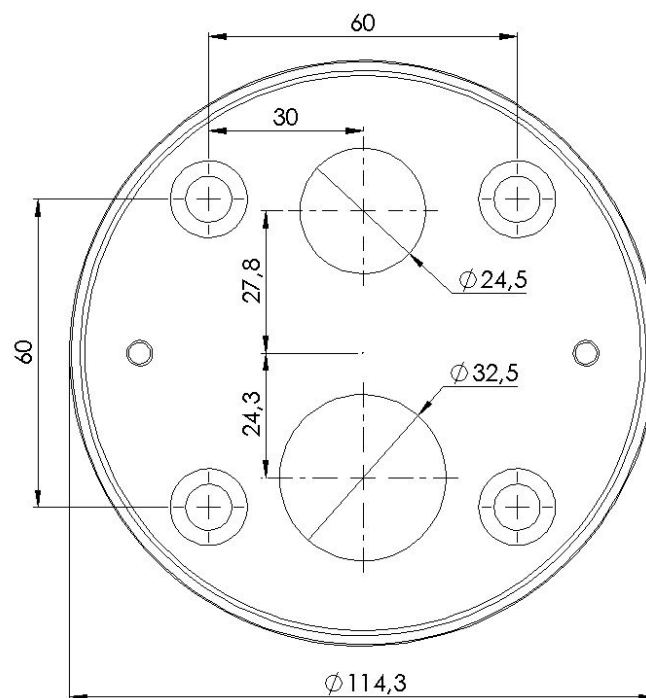
Abmessungen Befestigungspunkte (Maßeinheit mm)
